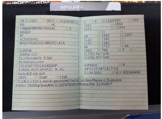
Abbildung 20: Fahrzeugdokumente
