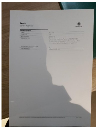
Abbildung 25: Fahrzeugdokumente
