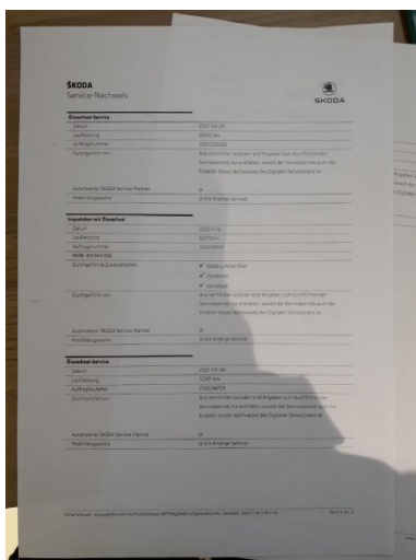
Abbildung 23: Fahrzeugdokumente
