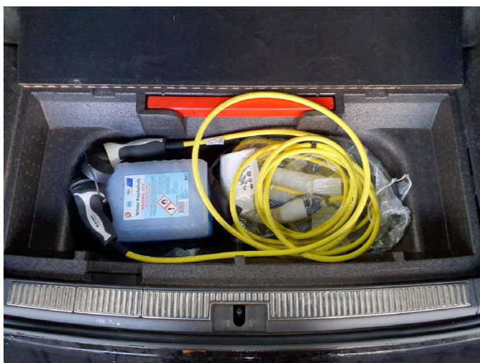
Abbildung 17: Zusatzausstattung
