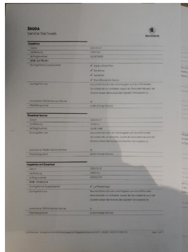
Abbildung 22: Fahrzeugdokumente
